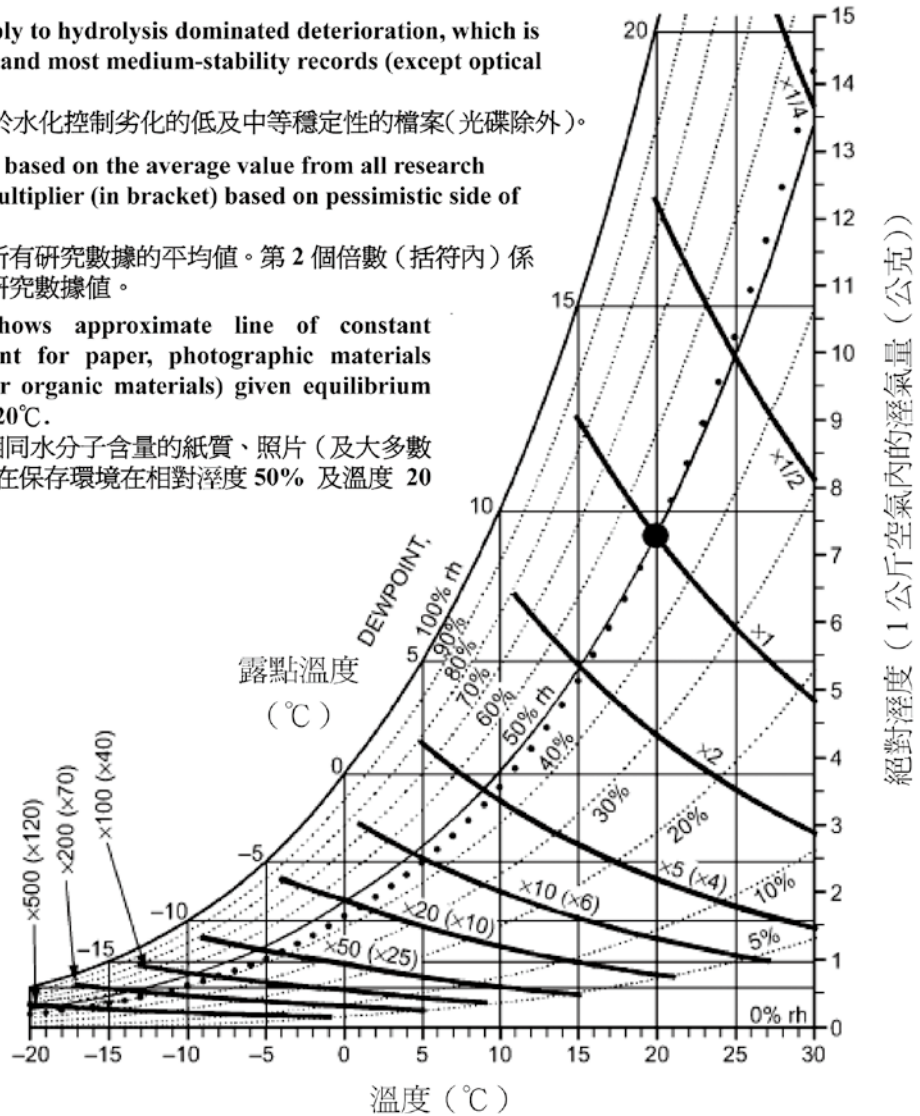
圖 26 不同溫度及相對溼度保存環境，相對於溫度 20°C 及相對溼度 (rh) 50% 之保存壽命倍數 (Lifetime Multipliers) 曲線圖。(資料來源 ASHRAE Applications Handbook CHAPTER 21 )
