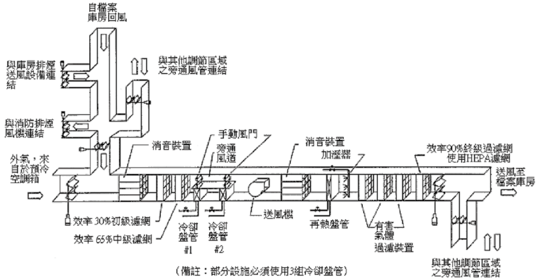
圖 35 美國國家檔案館 II 館之空調風管系統圖
